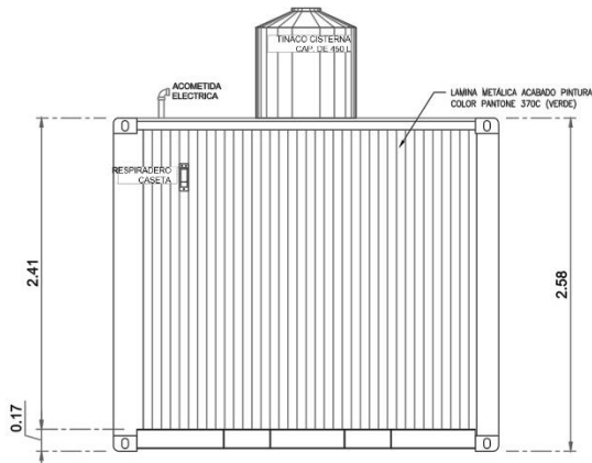
3 MODULO A VISTA POSTERIOR
