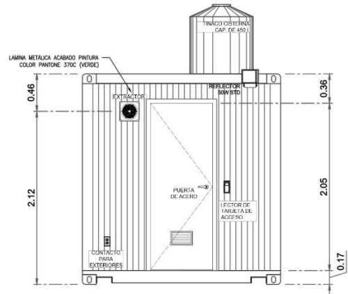
2 MODULO A VISTA LADO DERECHO
