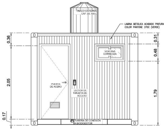
1 MODULO A VISTA FRONTAL
