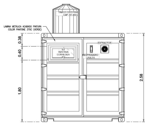
4 MODULO A VISTA LADO IZQUIERDO
